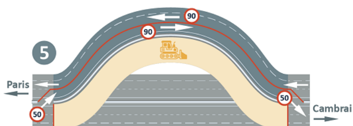
Phase 5 – Circulation du sens Paris/Cambrai sur la déviation provisoire
