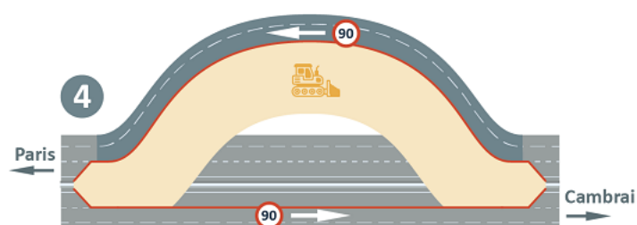
Phase 4 – Circulation du sens Cambrai/Paris sur la déviation provisoire
