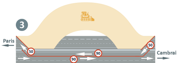
Phase 3 – Raccordement de la déviation à l'A2 sens Cambrai/Paris
