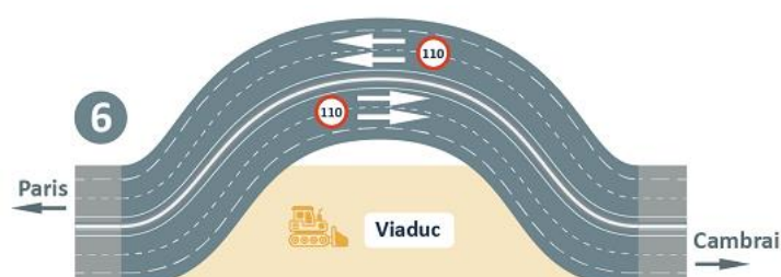
Phase 6 – Circulation sur la déviation provisoire pendant 2 ans et construction du viaduc
